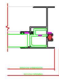
401 JAMB SERIES: 3500
